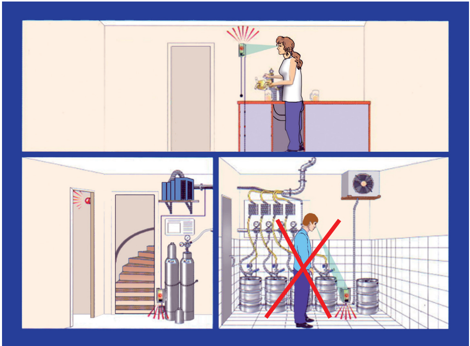
Abb. 10: Beispiel einer Installation einer Gaswarnanlage mit Sensoren für Kohlendioxid. Bei Hauptalarm ist das Betreten des Gefahrenbereichs (in diesem Fall der Keller) verboten!
